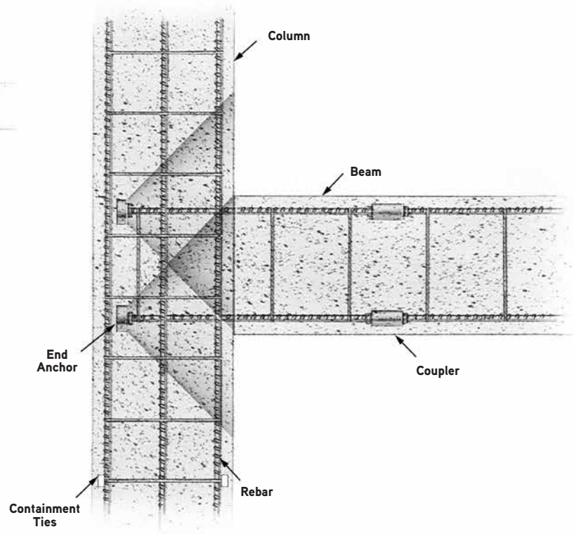
Elevation
