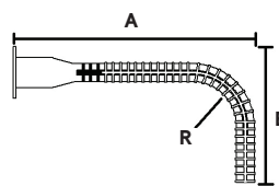
Type 2 90° Bend
