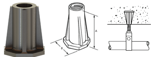
P86 Star Insert
