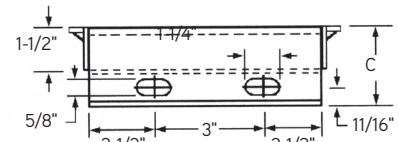
8" Insert
