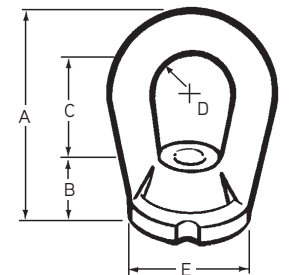
F48 Eye Nut
