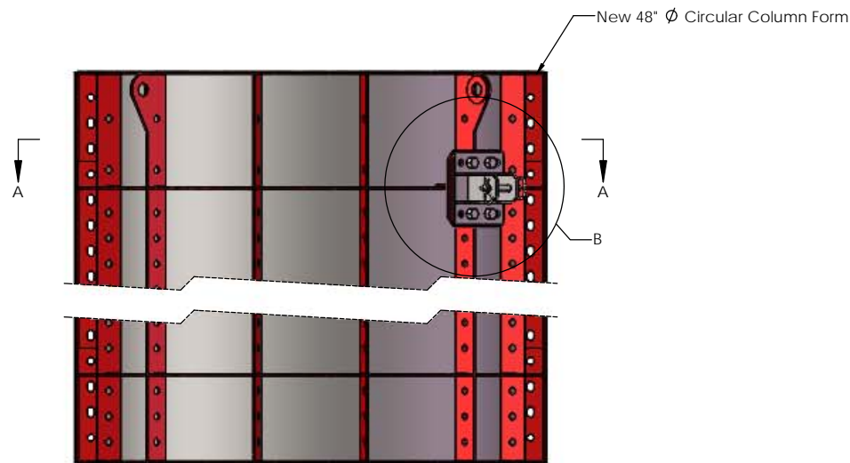
101 - ELEVATION
