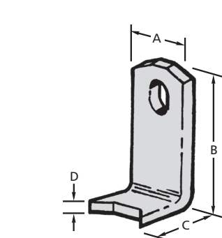
P93L L-ANCHOR
