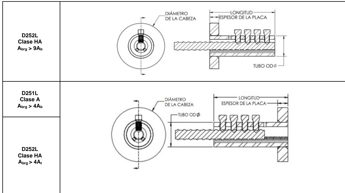
Figura 2 – Anclaje de Extremos Bar-Lock
