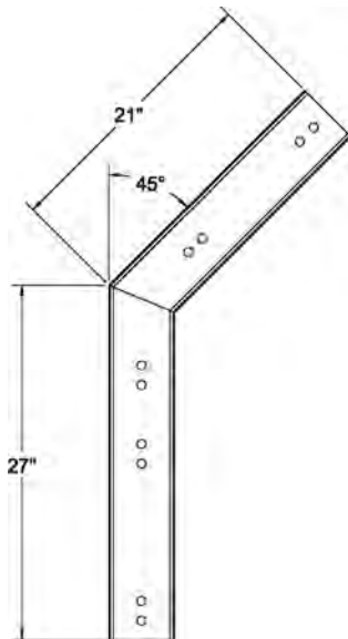
5" x 45° Waler
