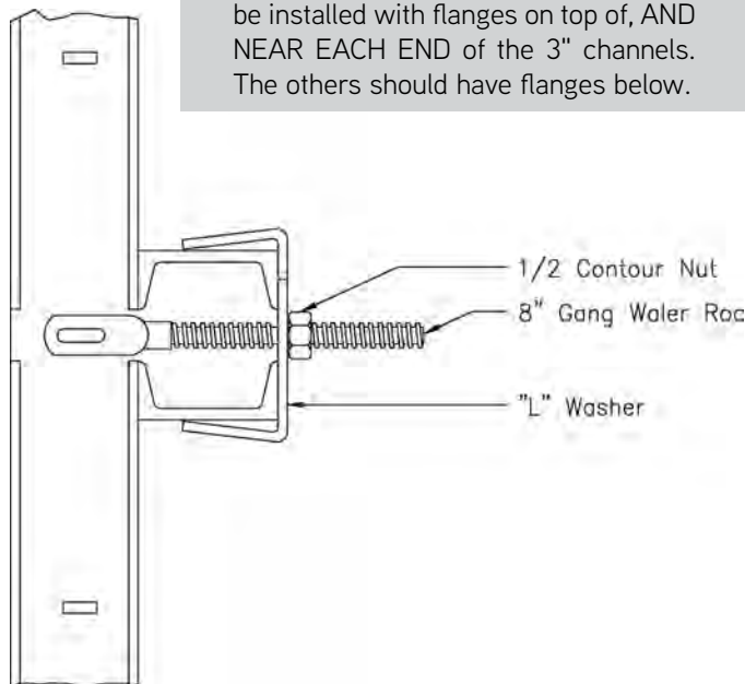
View A-A
