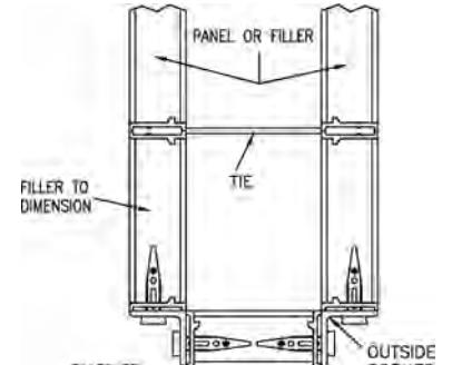
Filler Bulkhead
