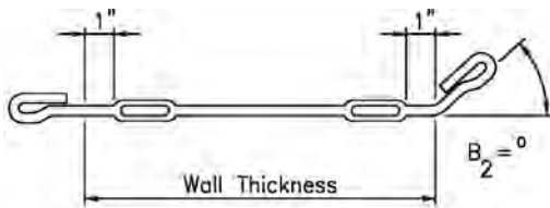
Pre-Bent Tie
